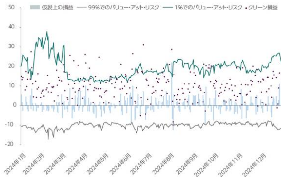
グラフ3：2024年におけるクレディ・アグリコル・CIBの規制バリュー・アット・リスクのバックテスト (単位：百万ユーロ)
