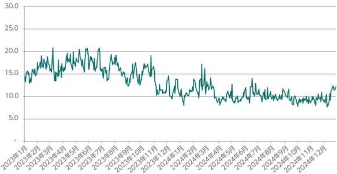
グラフ1：2023年 - 2024年の期間におけるクレディ・アグリコル・CIBの規制バリュー・アット・リスク (単位：百万ユーロ)
