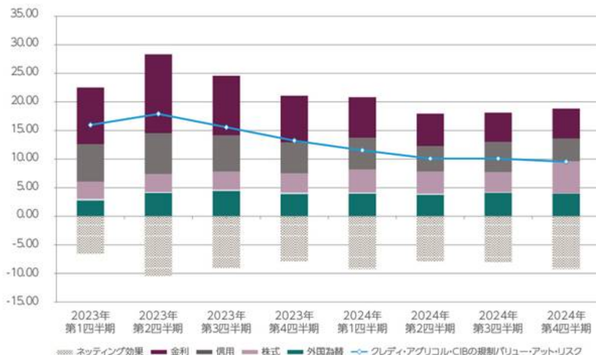
グラフ3：2024年におけるクレディ・アグリコル・CIBの規制バリュー・アット・リスクのバックテスト (単位：百万ユーロ)
